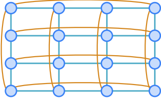
(d) çift simit 4×4 · çap 4
