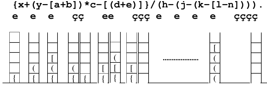
Şekil 5.1 : İfadelerin parantez geçerliliğinin belirlenmesinde kullanılan yığıt
